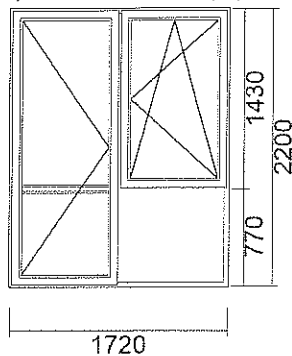
4) DRZWI BALK. 1-SK. (RL) 1720 x 2200
