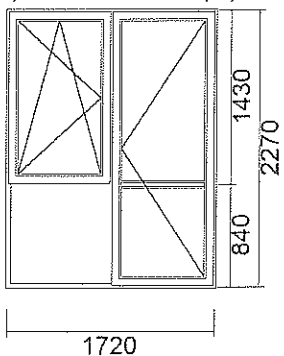
2) DRZWI BALK. 1-SK. (RL) 1720 x 2270
