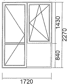
1) DRZWI BALK. 1-SK. (RL) 1720 x 2270
